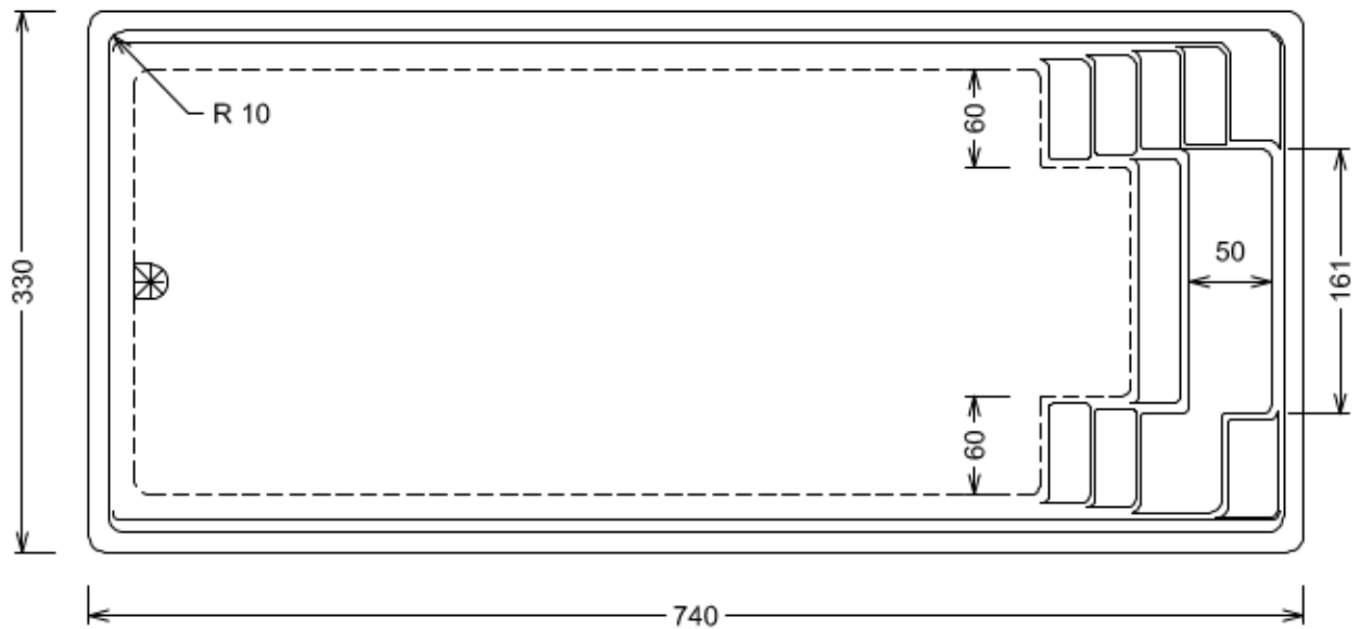
Grundriss - Pianta
