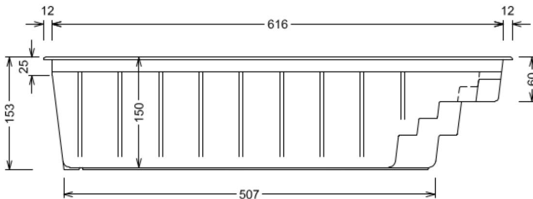
Seitenansicht - Prospetto laterale
