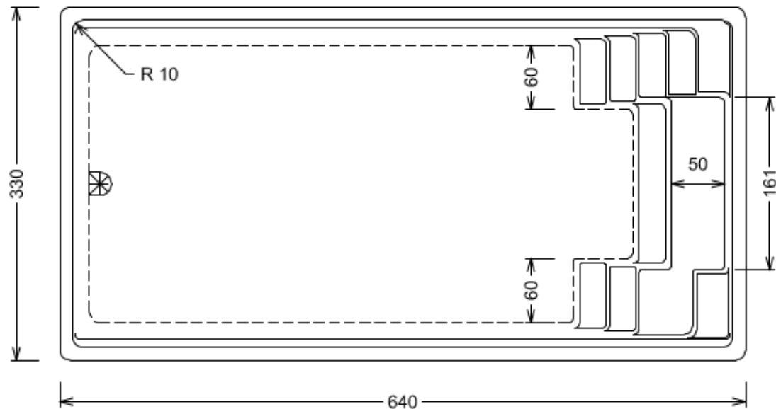
Grundriss - Pianta
