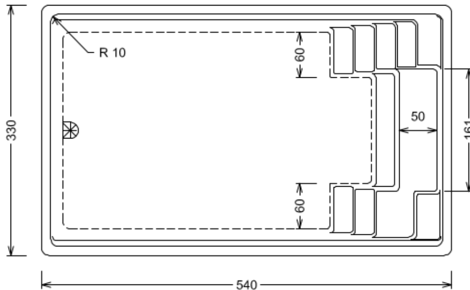
Grundriss - Pianta
