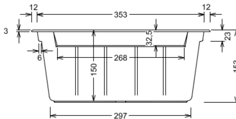
Ansicht Skimmerseite - Prospetto parte Skimmer
