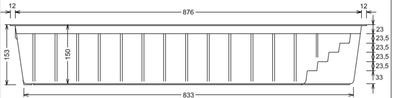
Seitenansicht - Prospetto laterale
